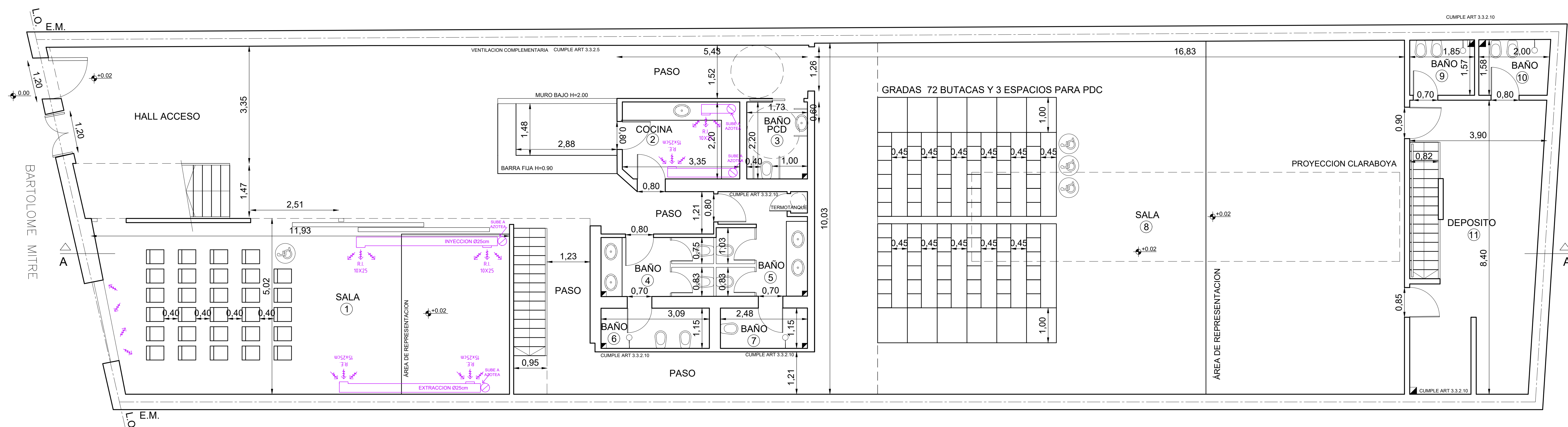
PLANTA BAJA
